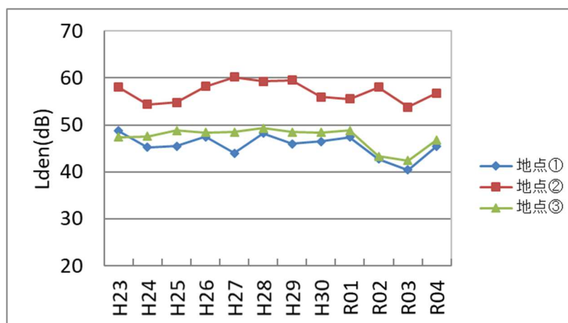
図2 経年変化(Lden)
