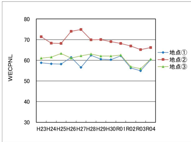
図3 経年変化(WECPNL)
